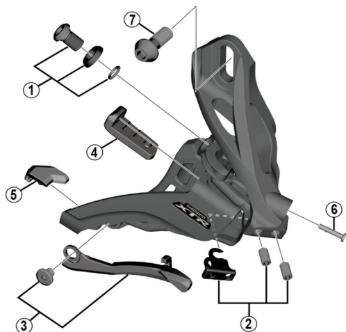
D-type
